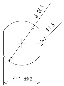
推奨取付穴形状
