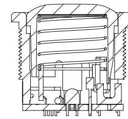
断面図 Z-Z
