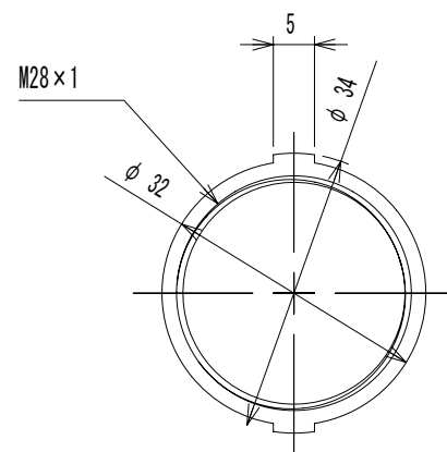
付属品 (固定ナット)
